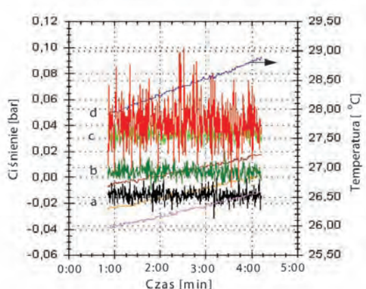
Rys. 6. Zmiany ciśnienia w strefie kawitacji i temperatury skawitowanej cieczy przy ciśnieniu zasilania: a) 6 bar, b) 7 bar, c) 8 bar, d) 9 bar, tarcza nr 3
