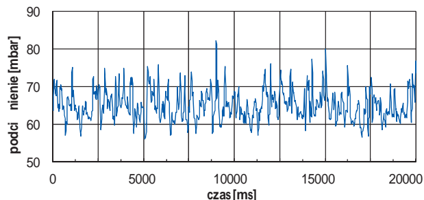
Rys. 5. Pulsacja ciśnienia w odległości ok. 45 mm od wzбудnika kawitacji
