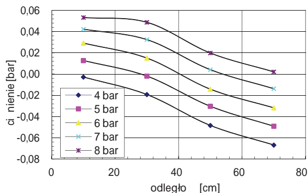
Rys. 7. Zmiany ciśnienia po stronie rozprężnej kawatatora w funkcji odległości od kryzy kawitacyjnej dla tarczy nr 3 i ciśnienia zasilania
