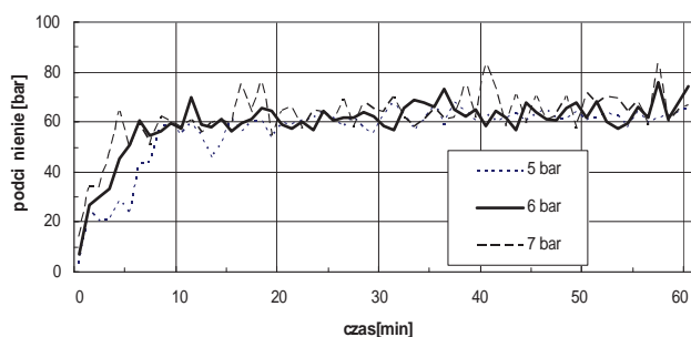
Rys. 4. Zmiany ciśnienia w strefie kawitacji w trakcie trwania okresu kawitacji dla tarczy nr 3
