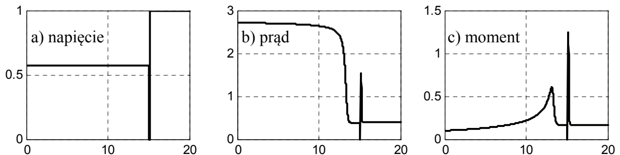
Rys. 13. Symulowane przebiegi napięcia, prądu obciążenia, momentu elektromagnetycznego. Oś rzędnych wyrażona w wartościach względnych, oś odciętych w sekundach
