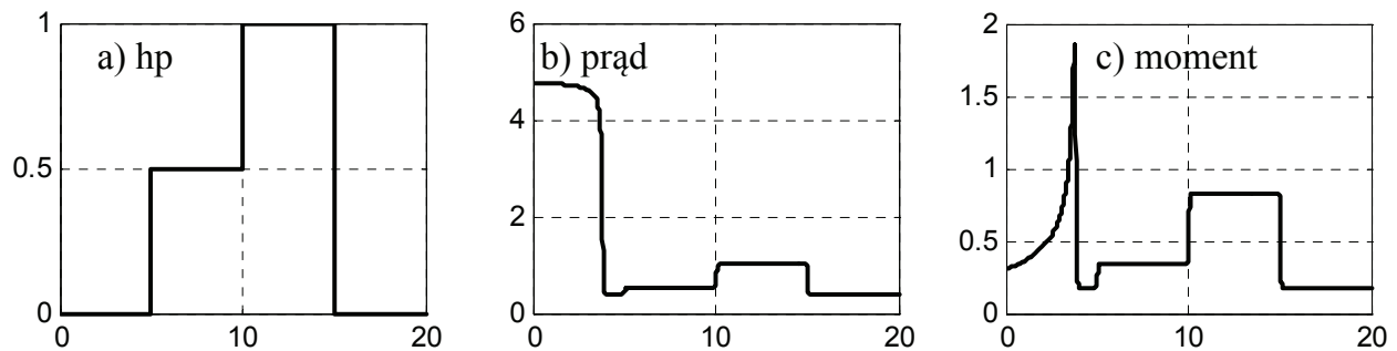
Rys. 12. Symulowane przebiegi skoku śruby, prądu obciążenia, momentu elektromagnetycznego. Oś rzędnych wyrażona w wartościach względnych, oś odciętych w sekundach
