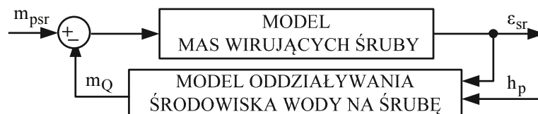
Rys. 8 – Struktura modelu śruby o zmiennym skoku
